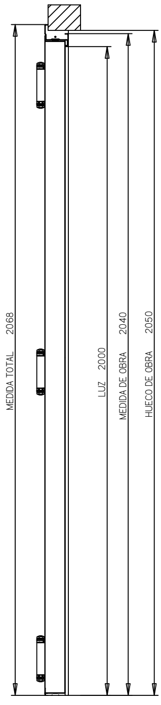
CORTE A-A 1:5
