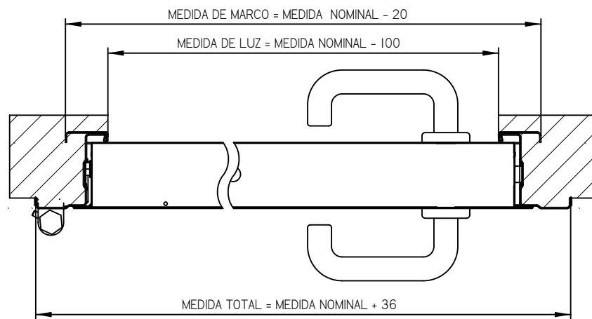
CORTE A-A
